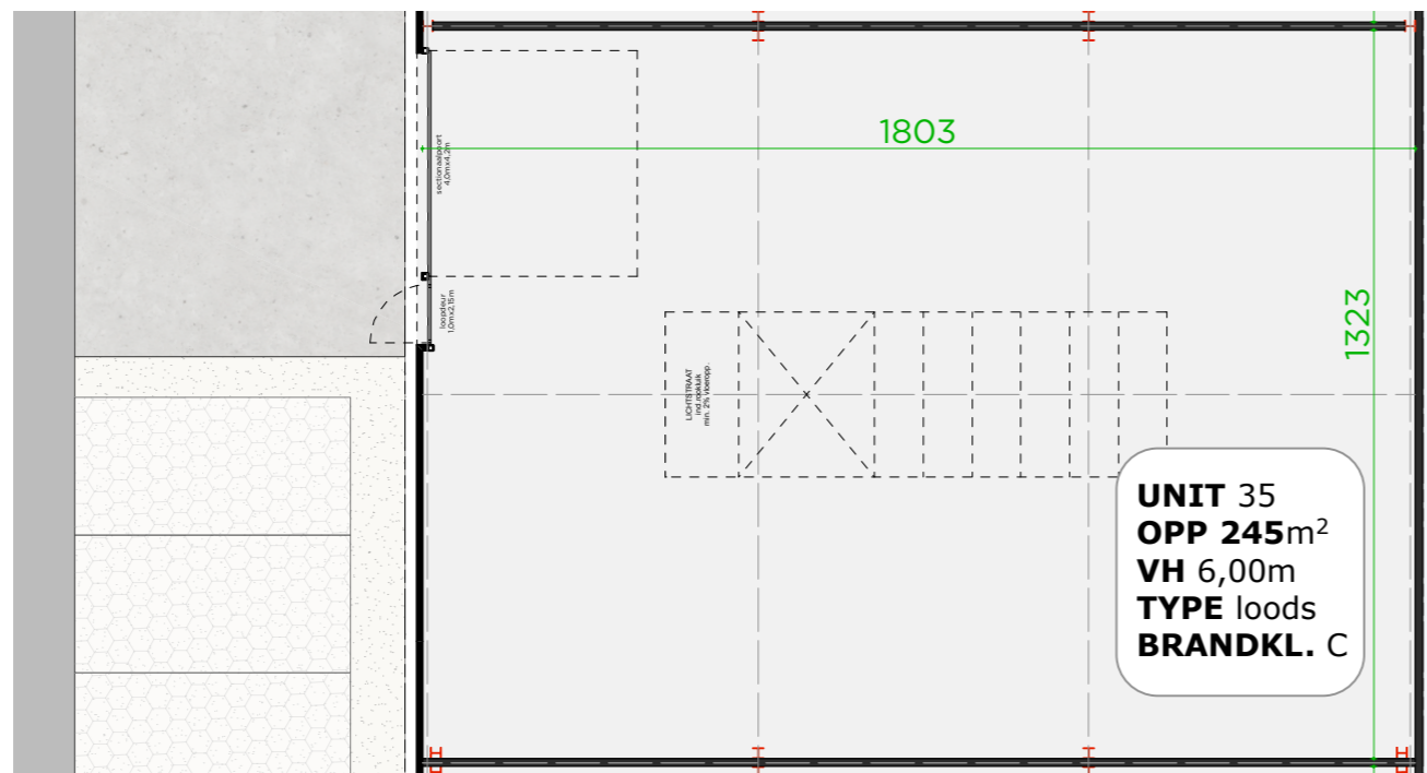
Grondplan
