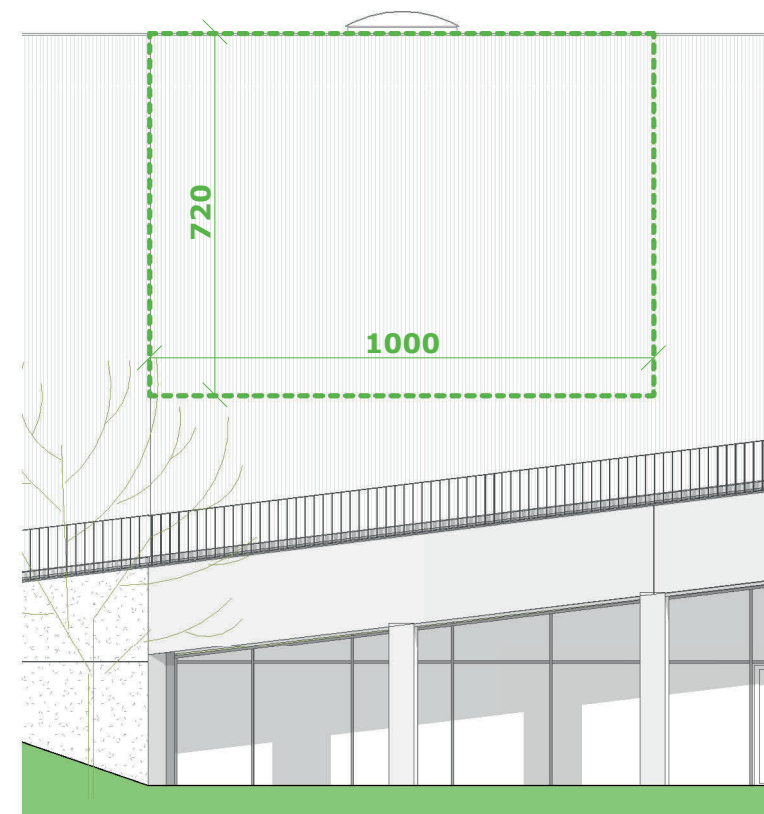
Zuidgevel
