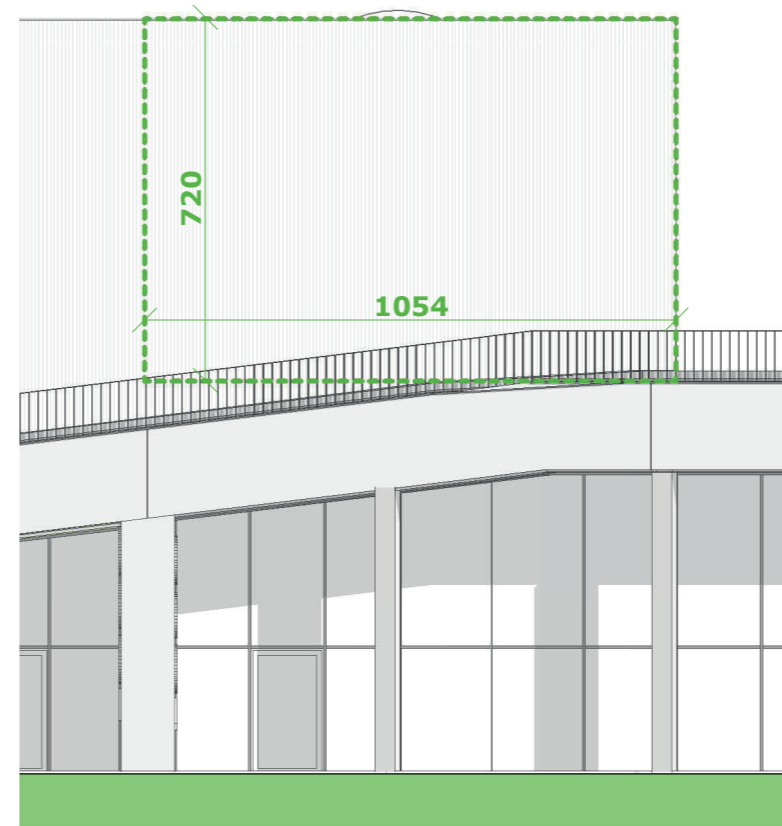
Zuidgevel
