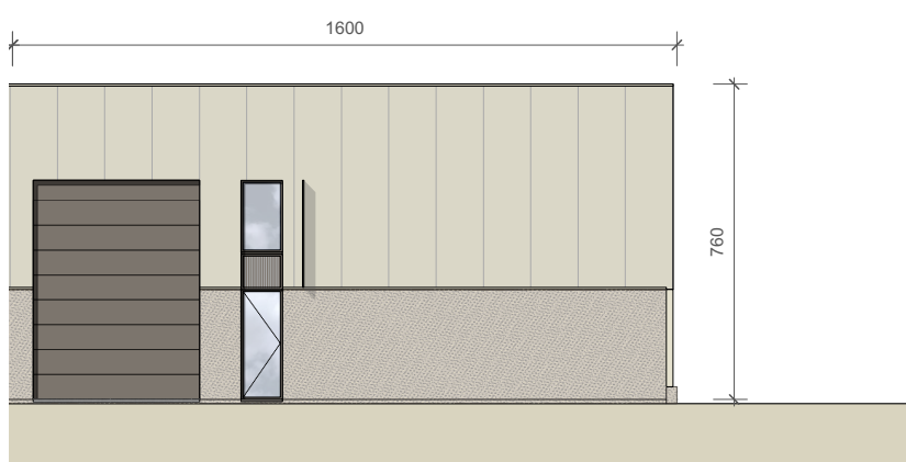
VOORGEVEL
