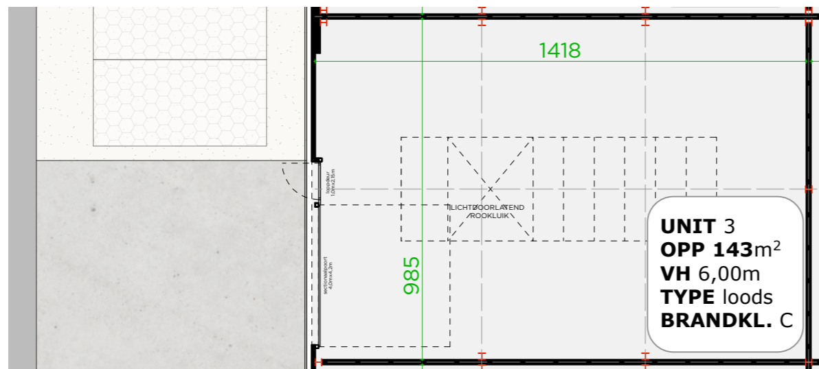
Grondplan
