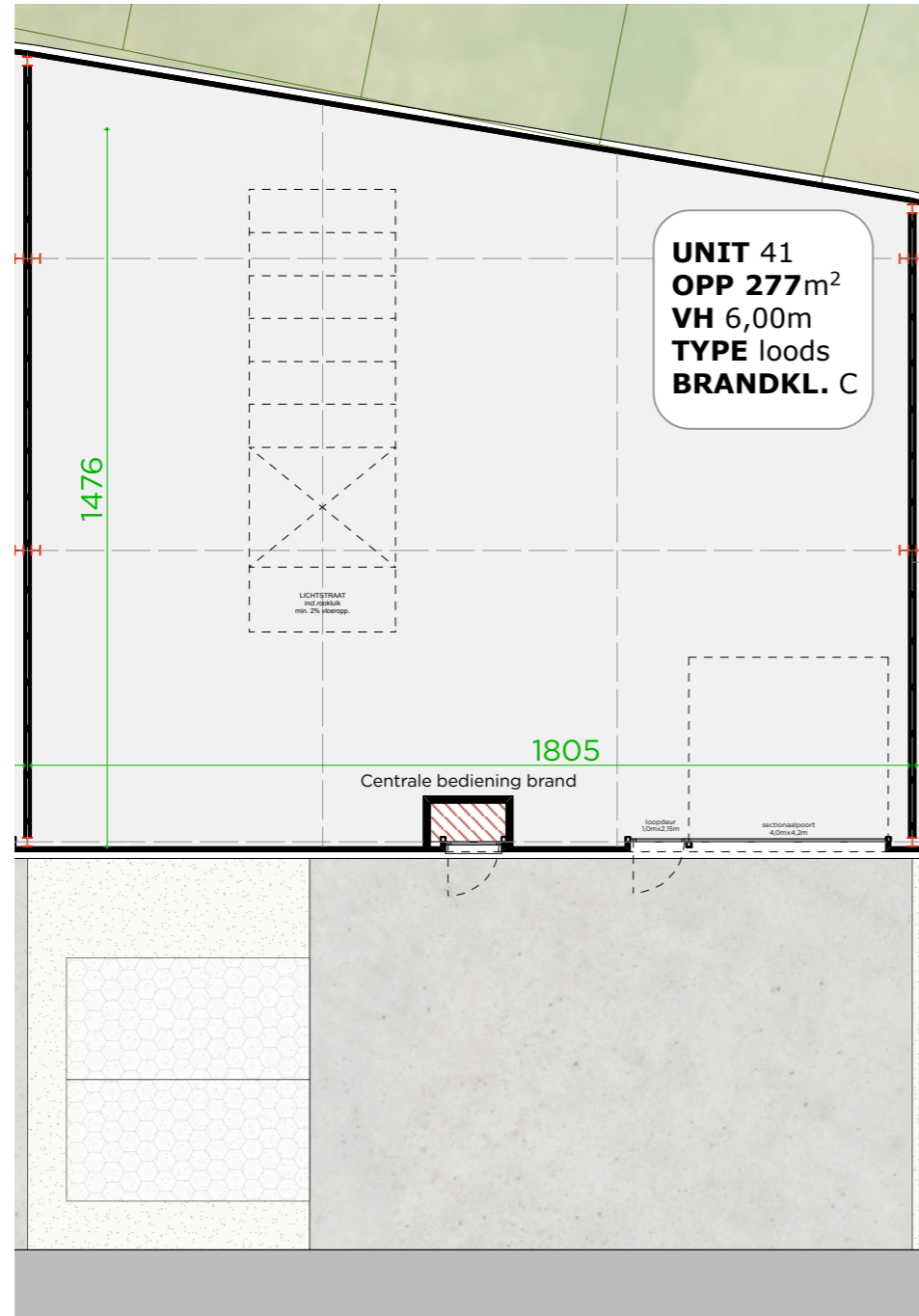
Grondplan
