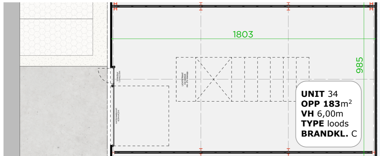
Grondplan
