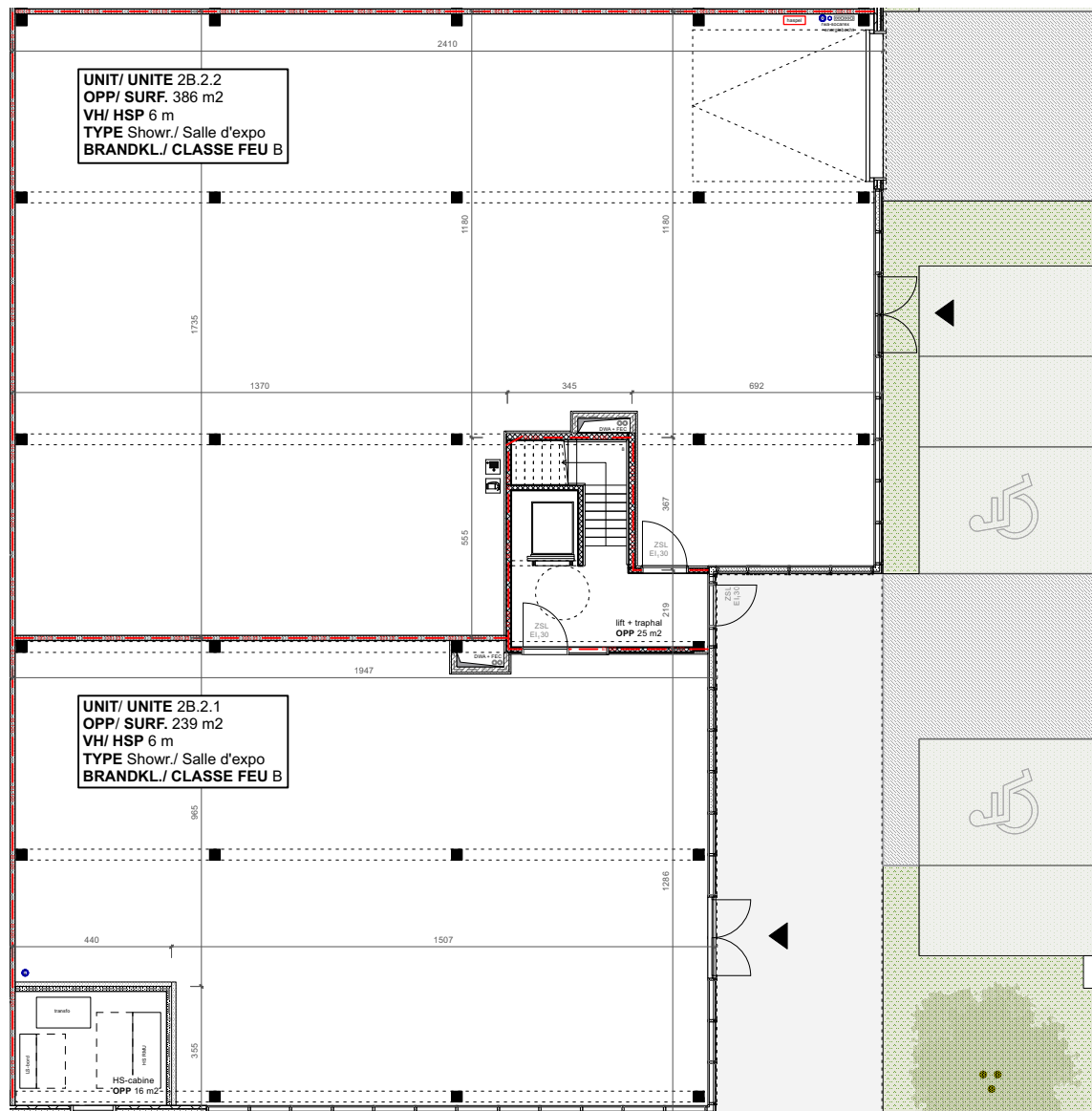
PLAN 0 - unit 2B.2.1 en 2B.2.2
